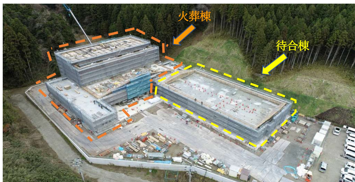
工事現場の様子（令和2年11月30日撮影）
